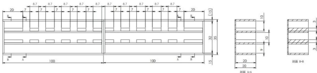
图4 物流分拣台
